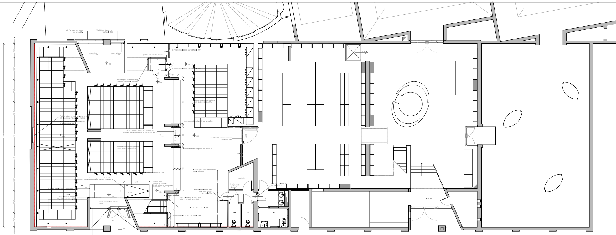
pianta a quota + 1.82
