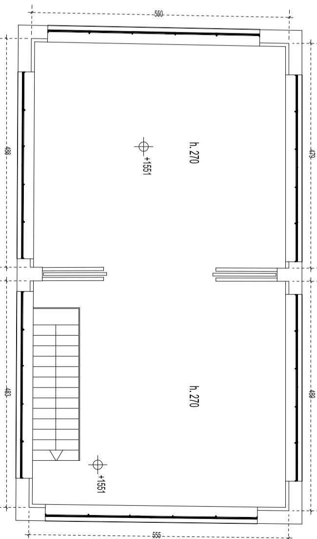
PIANO PRIMO
